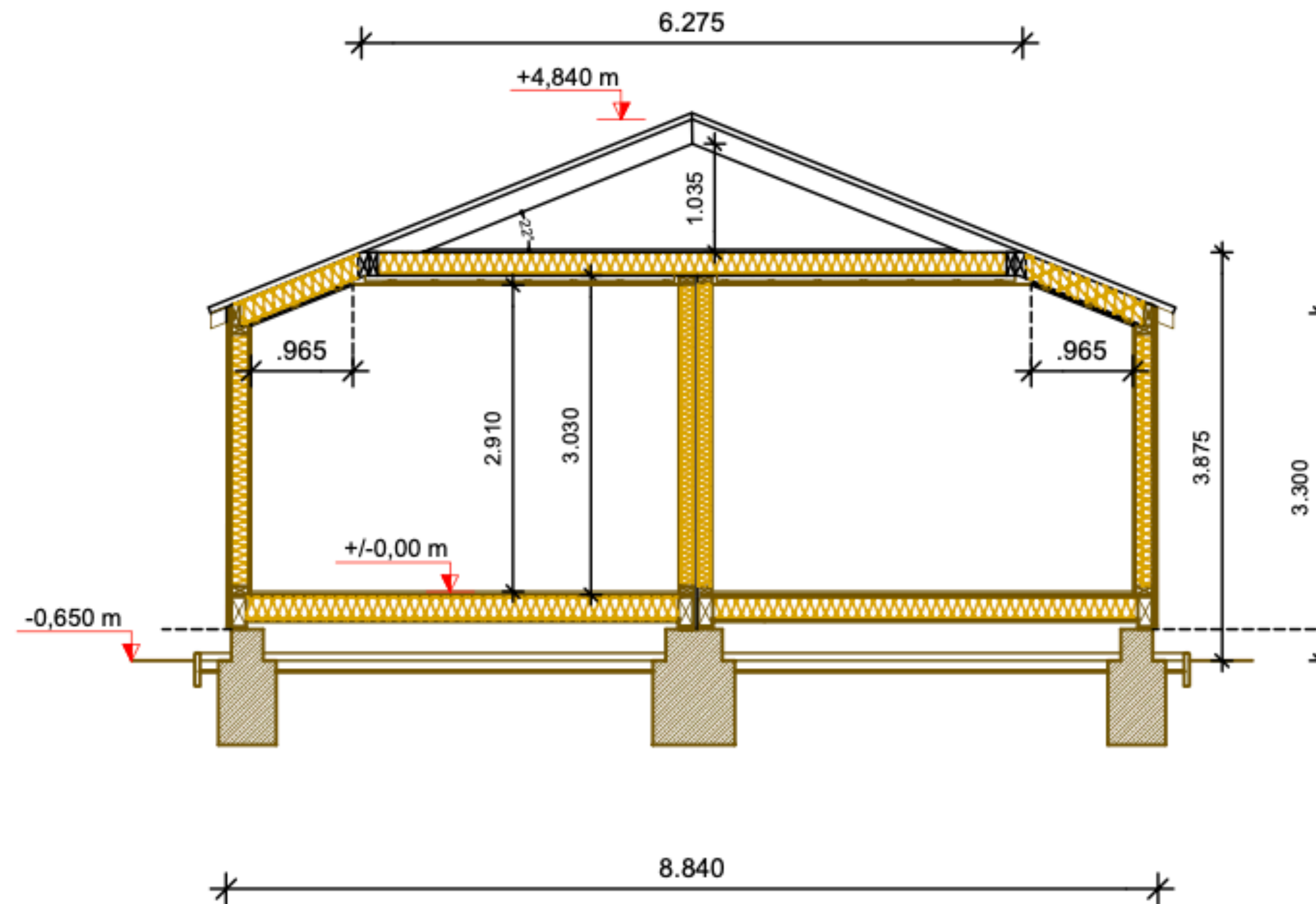
Schnitt M 1:100
